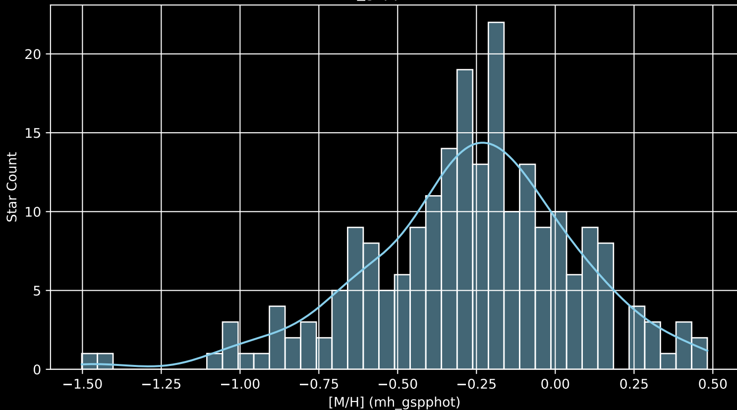
APOGEE DR17 Field: [283+67_btx [M/H] (mh_gspphot) (n= 218)
