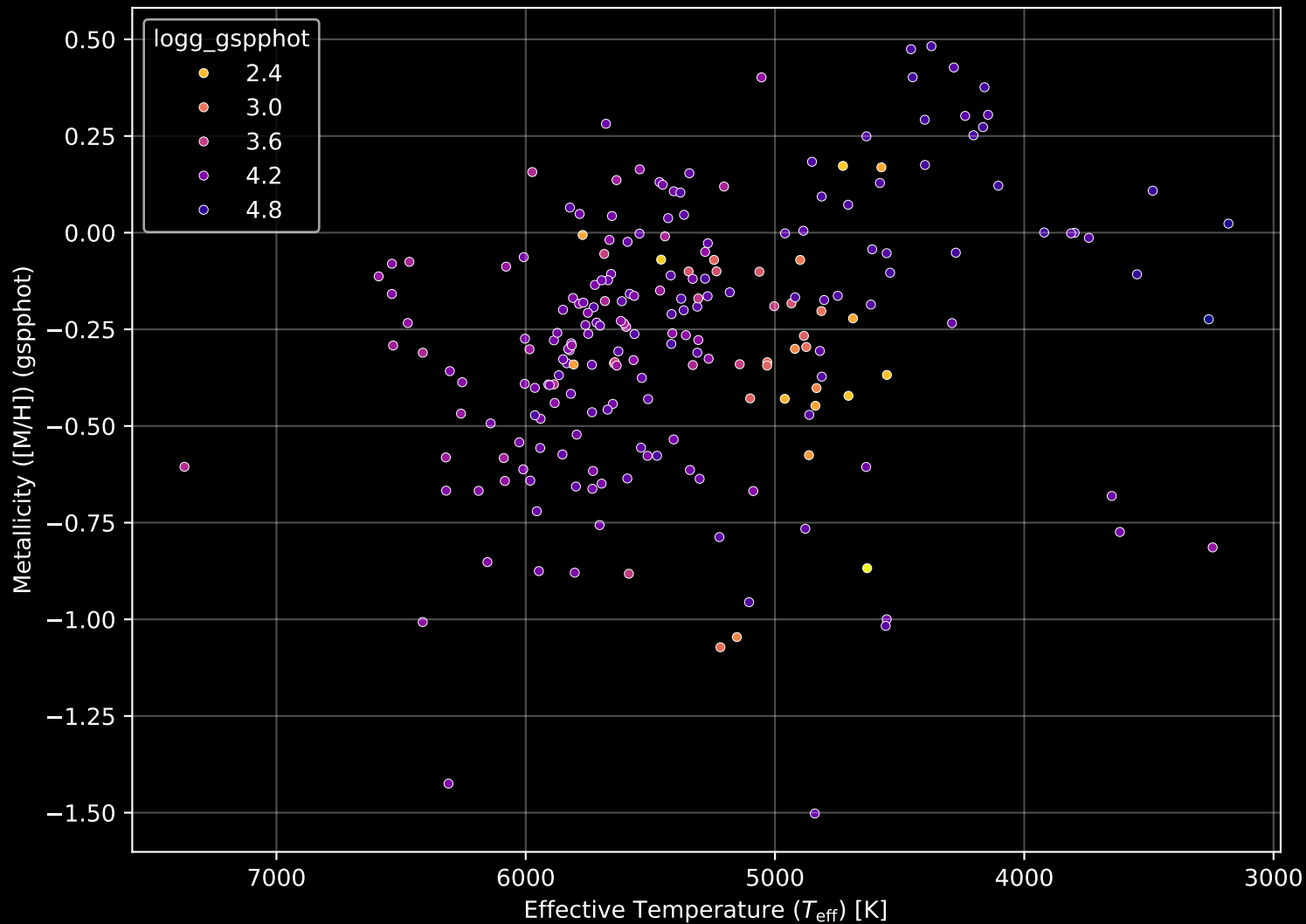
APOGEE DR17 Field: [283+67_bt] Stellar Population Parameters (n= 218)
